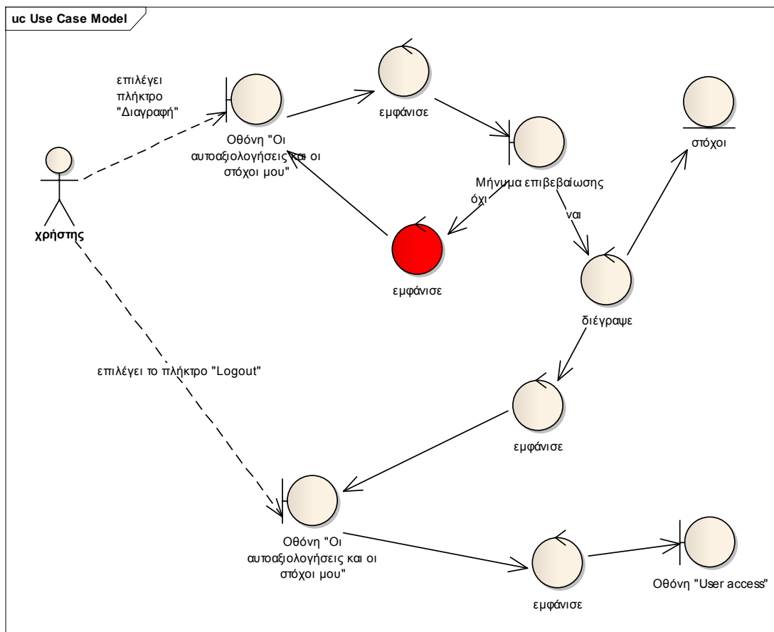
Διάγραμμα 21: Διάγραμμα ευρωστίας (robustness diagram) Διαγραφή στόχων
